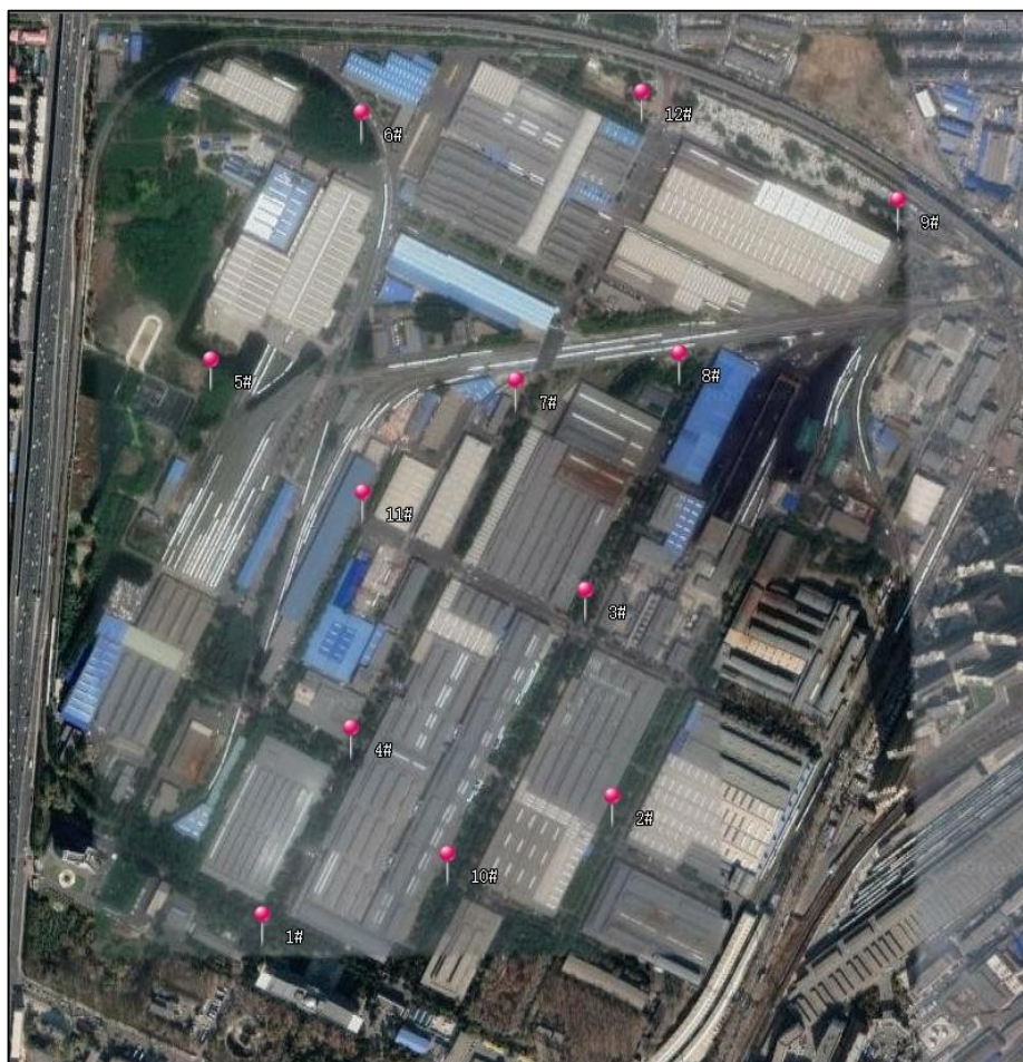
图17 老厂区土壤监测点位分布图
