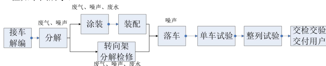
图 6 检修车总体工艺流程示意图
