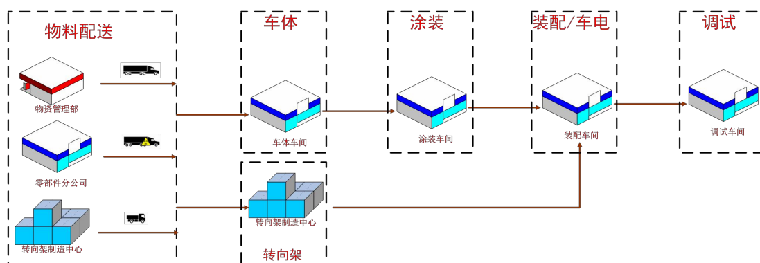
图 3 新造车生产流程示意图
