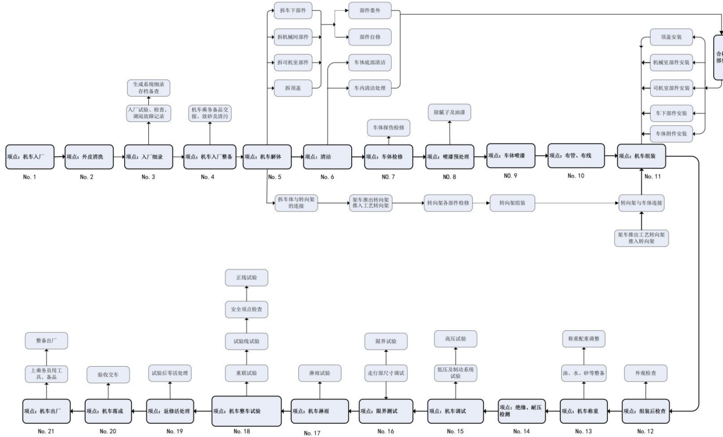
机车C6修工艺流程图
